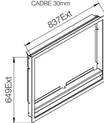
CADRE 30mm
